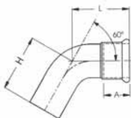
Curva 60° MF corta
