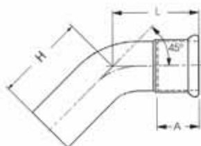
Curva 45° MF
