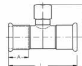
Tee con derivazione filettata femmina gas cilindrica
