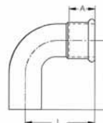
Curva 90° MF corta
