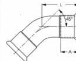
45° FF elbow
