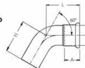
Curva stretta 60° M.F. R=1D
