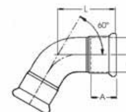
Curva stretta 60° F.F. R=1D
