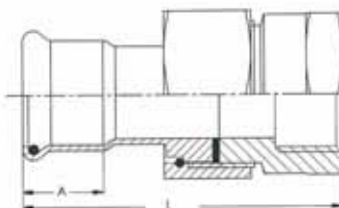
Bocchettone a sede piana attacco a pressare con filetto F cilindrico
