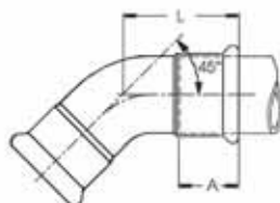
Curva stretta 45° F.F. R=1D
