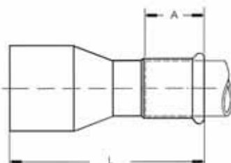
Riduzione concentrica
