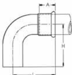
Curva stretta 90° M.F. R=1D
