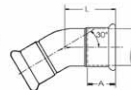
Curva stretta 30° F.F. R=1D
