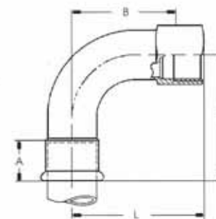
Curva mista 90° con filetto F gas cilindrico
