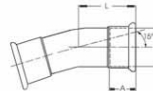
Curva 15° F.F. R=1,5D
