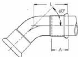
Curva 60° F.F. R=1,5D
