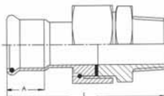
Bocchettone a sede piana attacco a pressare con filetto M conico
