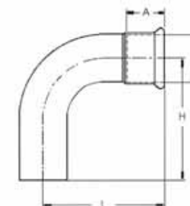
Curva 90° M.F. R=1,5D
