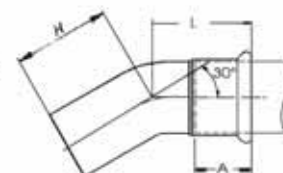
Curva stretta 30° M.F. R=1D
