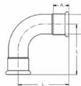
Curva 90° F.F. R=1,5D
