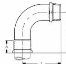
Curva mista 90° con filetto M gas conico
