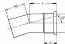
15° M.F. Elbow R=1,5D
